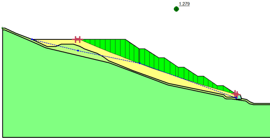
M-P 法 (fos=1.279)
