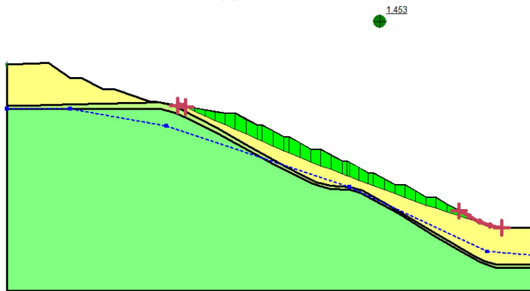
Sarma 法 (fos=1.453)
