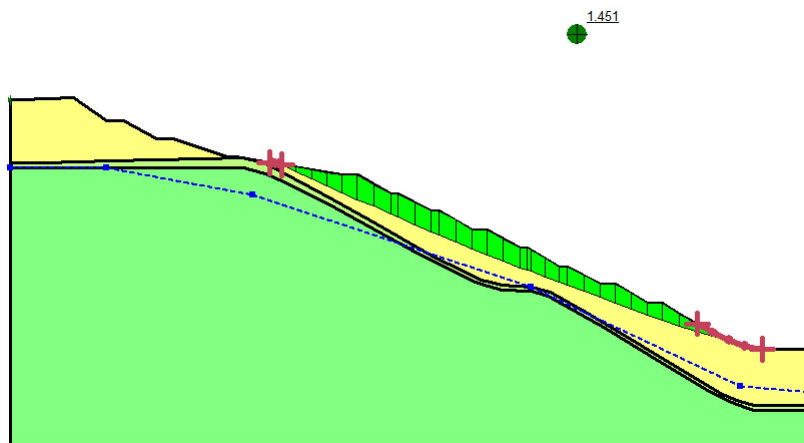
剩余推力法 (fos=1.451)
