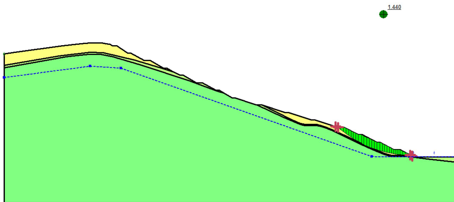
M-P 法 (fos=1.440)
