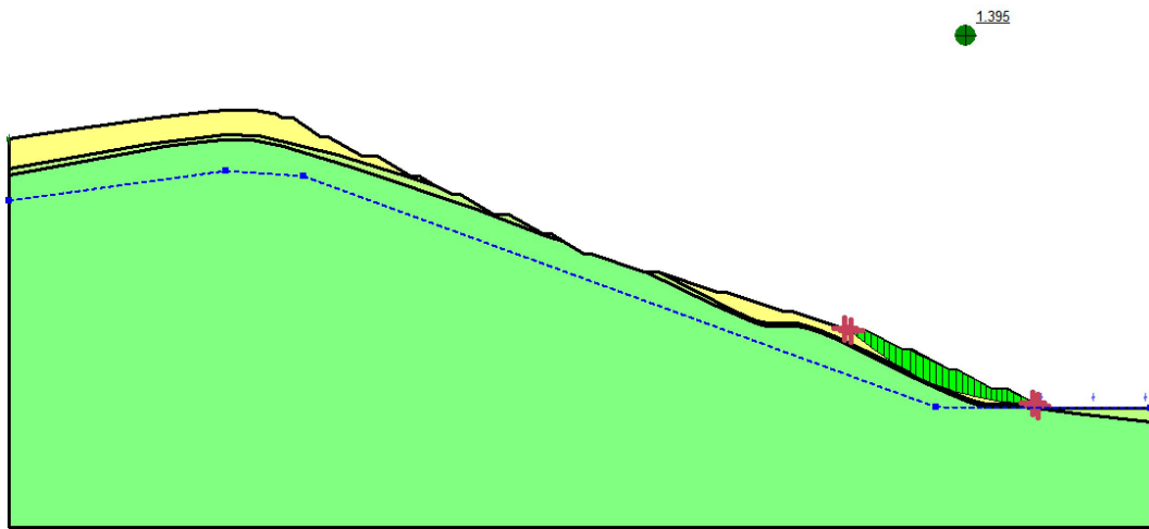
剩余推力法 (fos=1.395)
