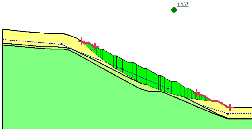
Sarma 法 (fos=1.157)
