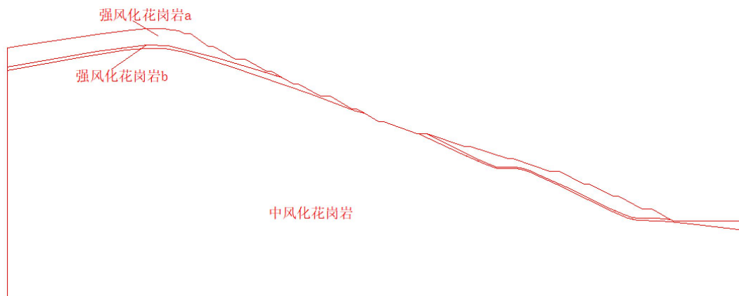
(a) 剖面 1-1’
