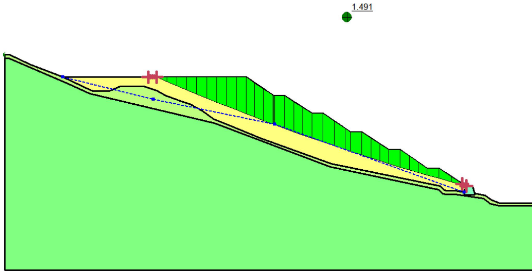
Sarma 法 (fos=1.491)
