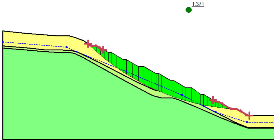
M-P 法 (fos=1.371)
