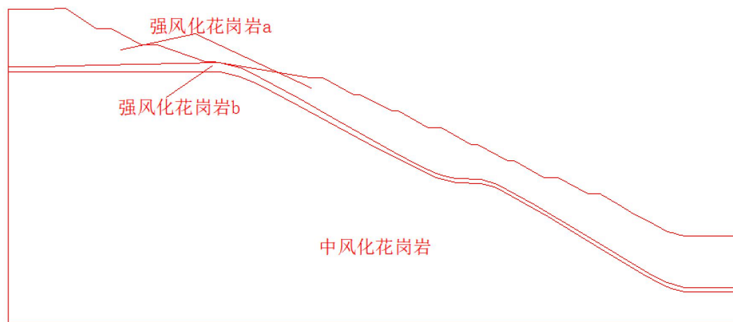
(b) 剖面 2-2’
