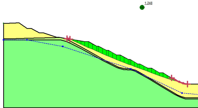
Sarma 法 (fos=1.248)
