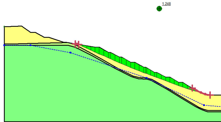
M-P 法 (fos=1.248)
