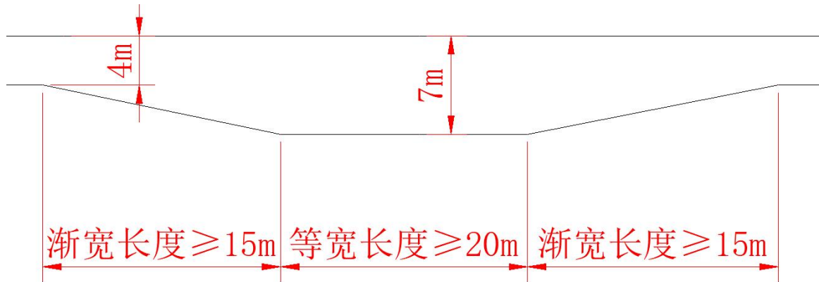
图 6.2-1 错车道图
