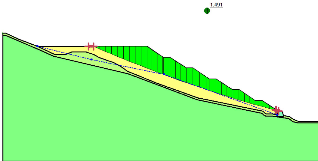
M-P 法 (fos=1.491)
