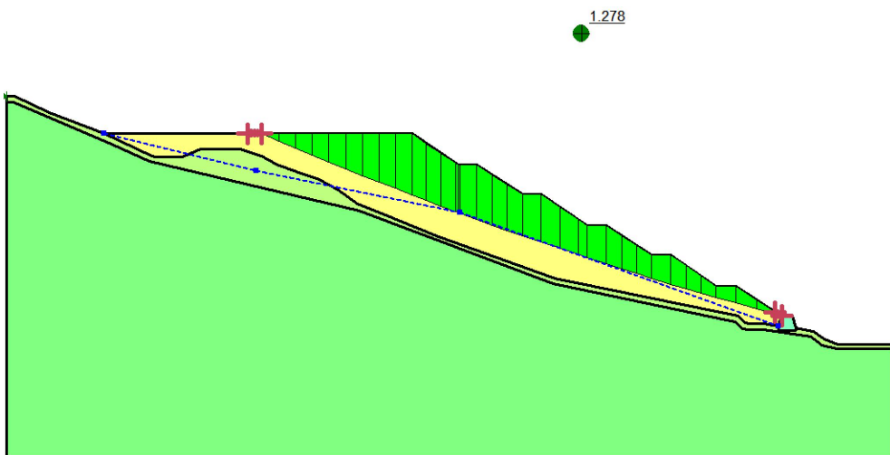
(c) 剩余推力法 (fos=1.278)
