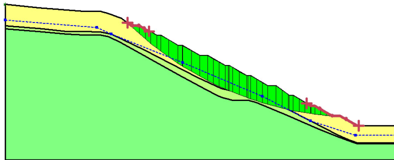
剩余推力法 (fos=1.187)
