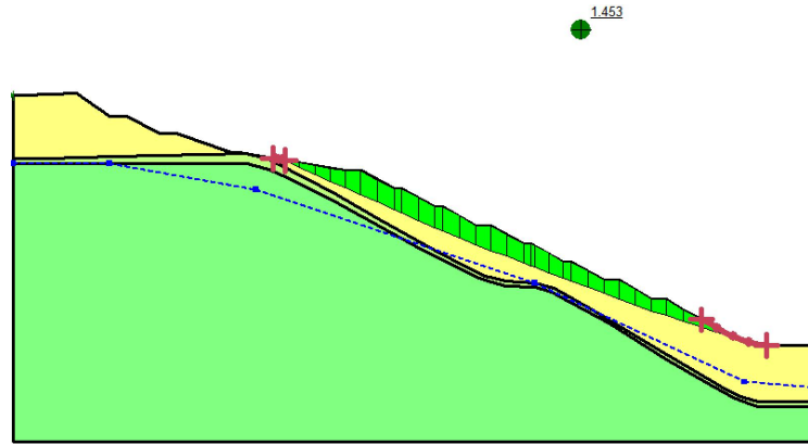
M-P 法 (fos=1.453)
