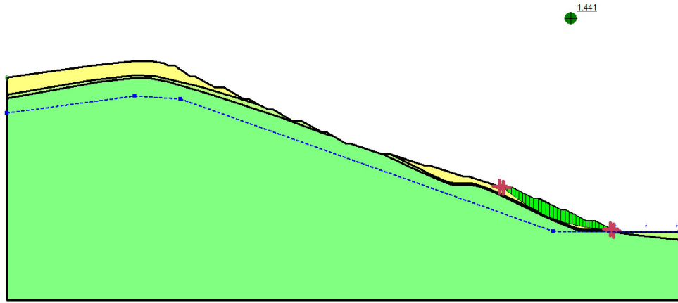
Sarma 法 (fos=1.441)
