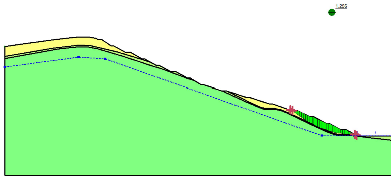
Sarma 法 (fos=1.256)
