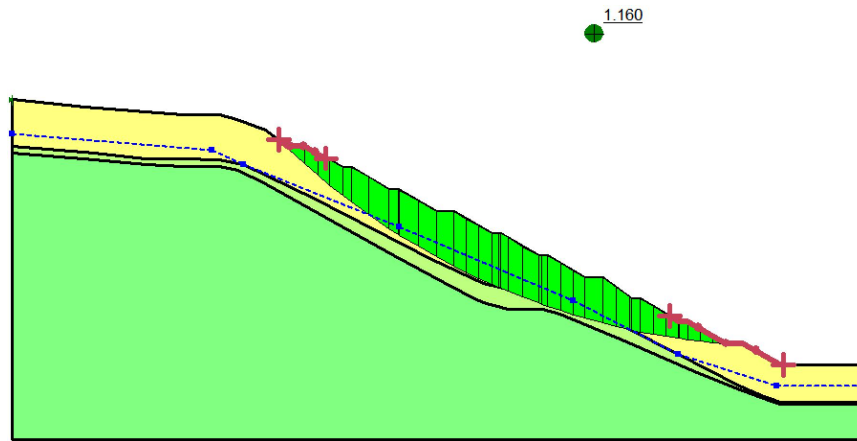
M-P 法 (fos=1.160)
