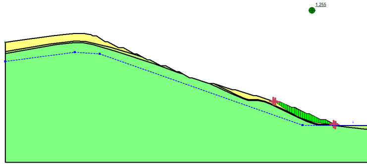
M-P 法 (fos=1.255)
