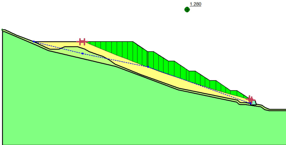
Sarma 法 (fos=1.280)
