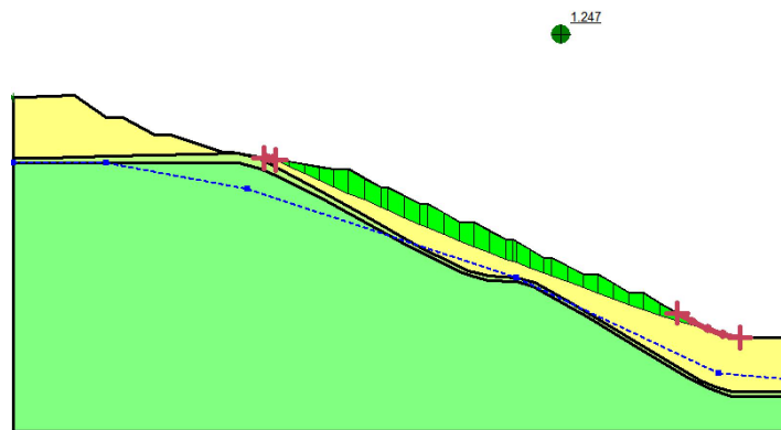
剩余推力法 (fos=1.247)
