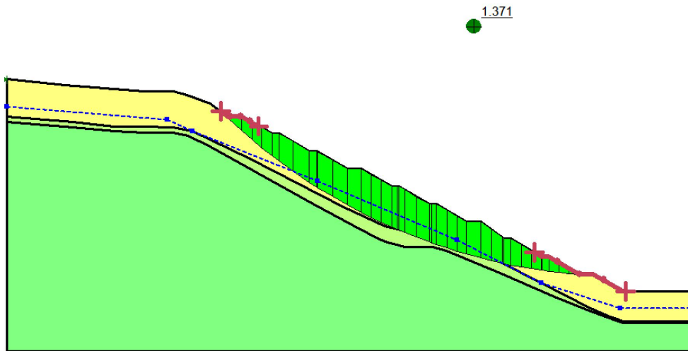
Sarma 法 (fos=1.371)
