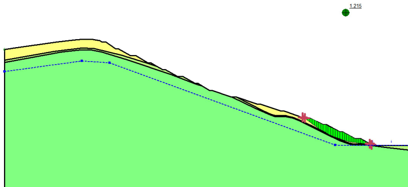
剩余推力法 (fos=1.215)
